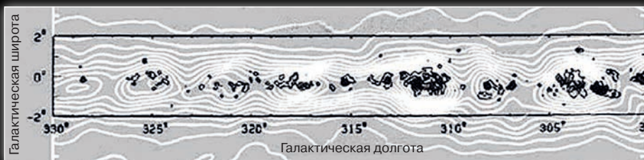
Сверхоблака HI (светлые контуры), внутри них — облака молекулярного водорода в отрезке рукава Киль. Указаны галактические долготы и широты.
