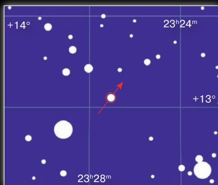
Оккультация звезды HIP 115751 ( \alpha = 23^h 27^m 04^s , \delta = 13^\circ 06' 38'' ) астероидом Вината (2347 Vinata) 8-9 августа
