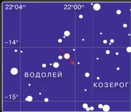
Оккультация звезды HIP 108649 ( \alpha = 22^{\text{h}}00^{\text{m}}39^{\text{s}} , \delta = -14^{\circ}09'52'' ) астероидом №5977 (1992 TH1) 20 августа
