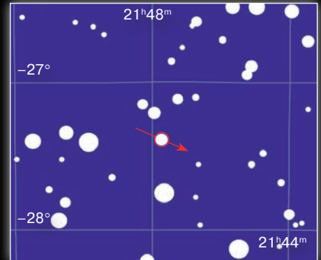
Оккультация звезды HIP 107613 ( \alpha = 21^{\text{h}}47^{\text{m}}46^{\text{s}} , \delta = -27^{\circ}23'13'' ) астероидом №7405 (1988 FF) 25-26 августа. Координаты звезд даны на эпоху 2000.0. Детали явлений — в тексте
