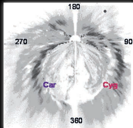
Регулярность расположения сверхоблаков HI вдоль рукавов Килья и Лебеда. Солнце находится в центре отсчета галактических долгот на расстоянии около 25 тыс. лет от центра Галактики
