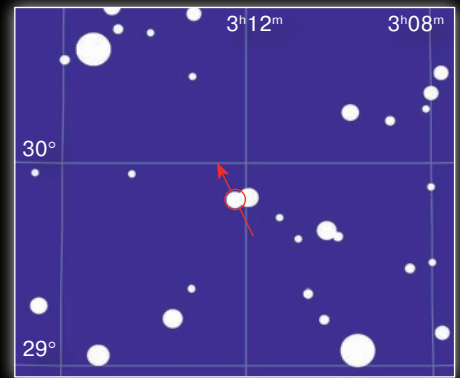
Оккультация звезды TYC 1795-455 ( \alpha = 3^{\text{h}}12^{\text{m}}16^{\text{s}} , \delta = 29^{\circ}49'07'' ) астероидом Илматар (385 Ilmatar) 24-25 августа
