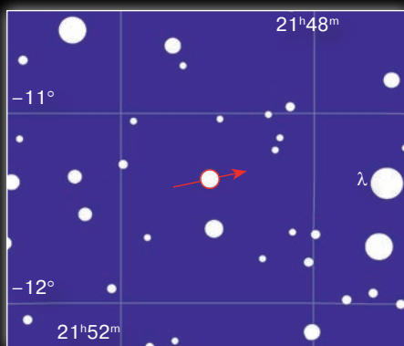
Оккультация звезды HIP 107793 ( \alpha = 21^h 50^m 11^s , \delta = -11^\circ 20' 35'' ) астероидом Люмен (141 Lumen) 11 августа
