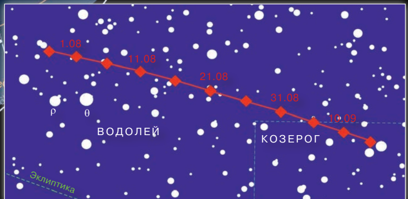
Видимый путь малой планеты Хигия (10 Hugia) в августе-сентябре 2012 г.
